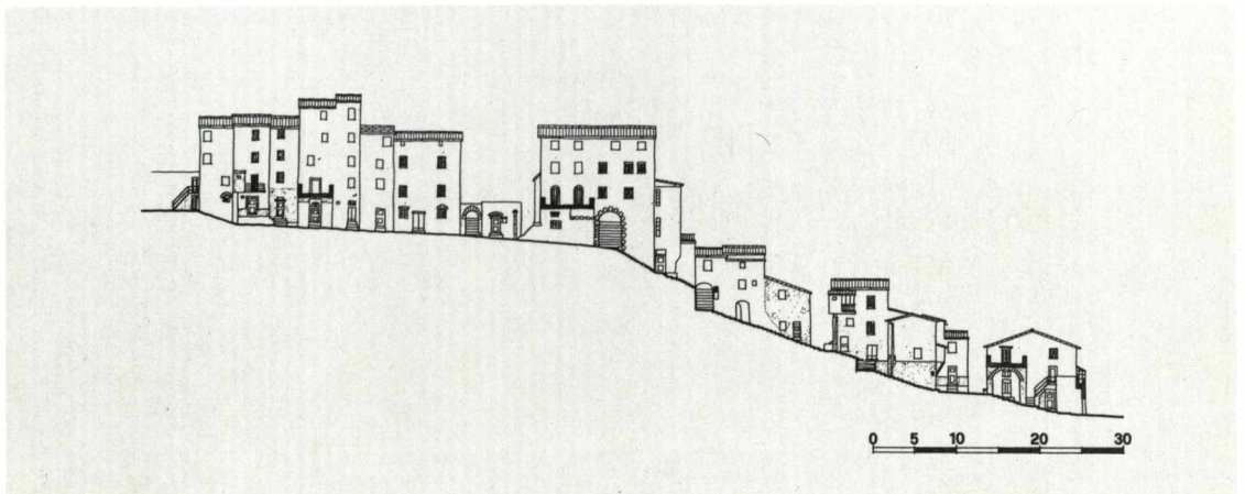
VEZZANO BASSO. Sezioni secondo la curva di livello e secondo la linea di massima pendenza rispettivamente; in entrambe evidente l'aggregazione delle cellule edilizie per schiere continue a girone.
