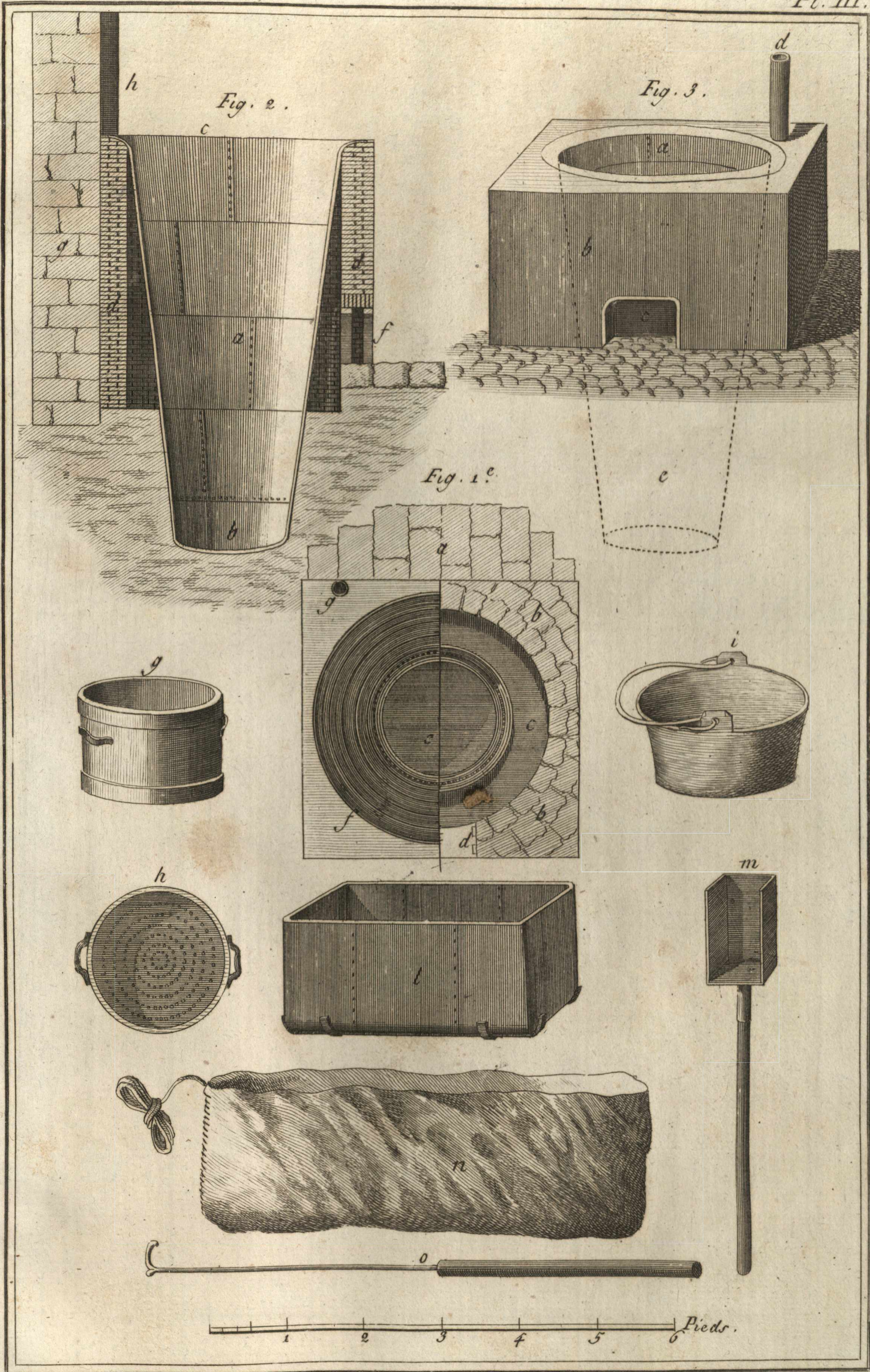
14 e Teinturier de Riviere, Plans, Coupe et Élevation de la Cuve pour l'Indigo. c
