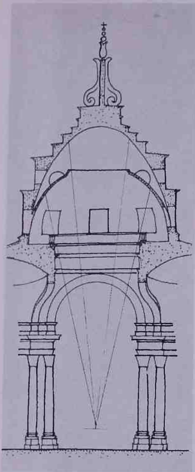
Fig. 4 - S. Gaetano di Vicenza (disegno dell'A., dall'«Architettura Civile» del Guarini).
