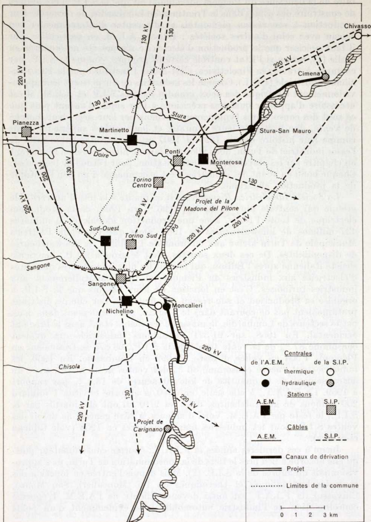
FIG. 6. — Stations et centrales électriques de l'agglomération de Turin
